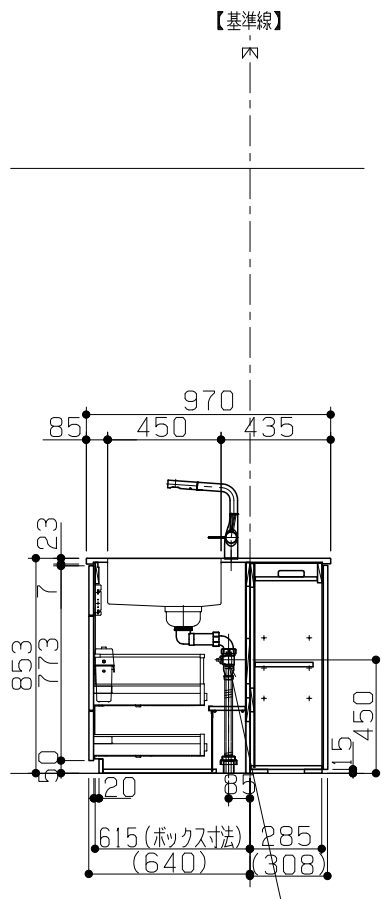
A-A 断面図
