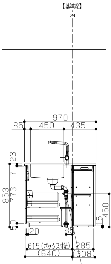
A-A 断面図
